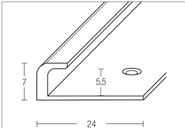
PVC-Abschlusskante Art.-Nr. Z 172
