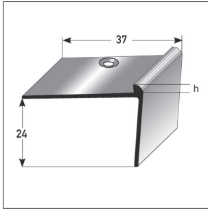
Step edge * Art.-Nr. Z 543
