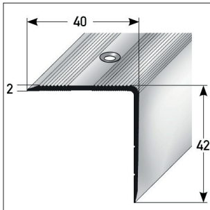
Angle edge 90° * Art.-Nr. Z 569
