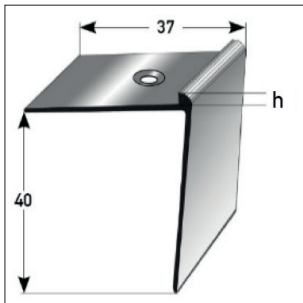
Step edge * Art.-Nr. Z 587
