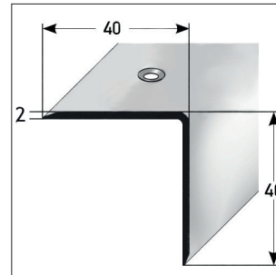
Platform profile/ Angle edge 90° * Art.-Nr. O 305
