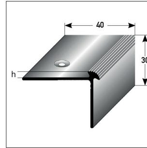
Step edge * Art.-Nr. Z 544
