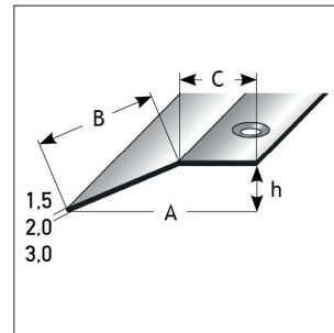
Anpassungsprofil Art.-Nr. Z 590
